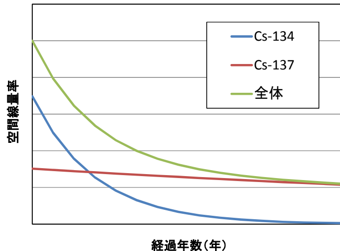
図2-67 Cs-134とCs-137の放射線量の減少
